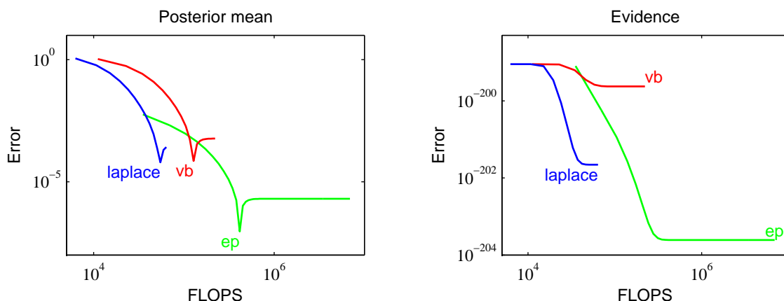
图 10.17: 期望传播、变分推断和拉普拉斯近似在聚类问题上的对比。左图给出了预测后验概率分布的均值与浮点运算的数量关系，右图给出了对应的模型证据的结果。
