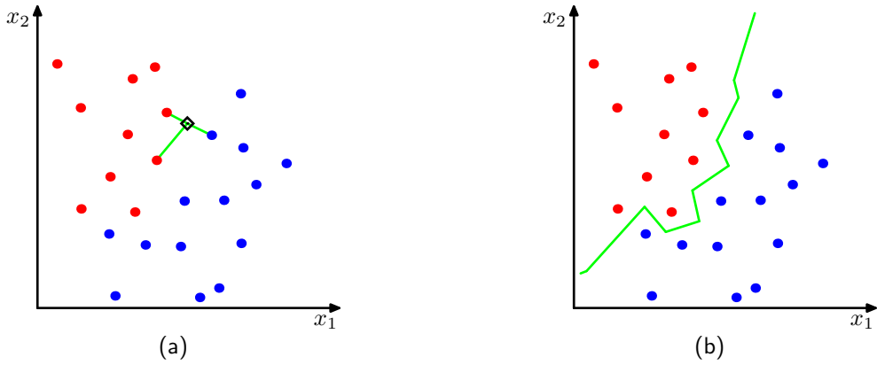
图 2.27: (a)在 K 近邻分类器中, 一个新的数据点(黑色菱形表示)根据 K 个距离最近的训练数据点的主要类别确定, 其中 K = 3 。(b)在最近邻( K = 1 )分类方法中, 生成的决策边界由不同类别的点对的垂直平分线组成的超平面确定。
