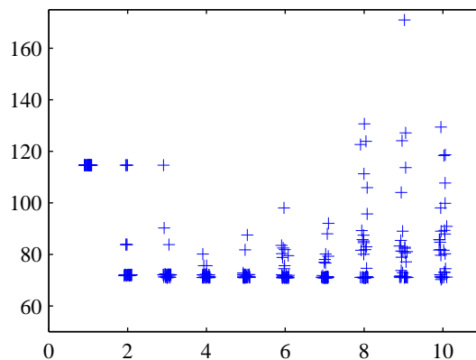
图 5.10: 对于多项式数据集，测试集的平方和误差与网络的隐含单元的数量图像的。对于每个网络规模，都随机选择了30个初始点，这展示了局部最小值的效果。对于每个新的初始点，权向量通过从一个各向同性的高斯分布中取样，这个高斯分布的均值为零，方差为10。
