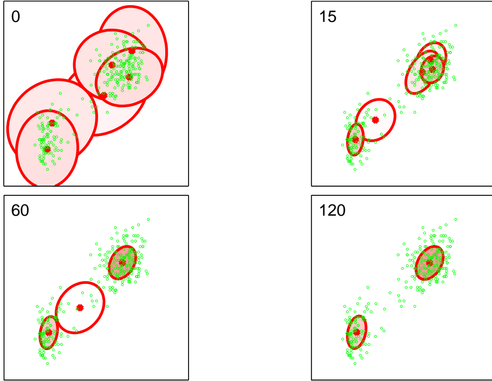
图 10.6: K = 6 个高斯分布的变分贝叶斯混合, 应用于老忠实间歇喷泉数据集, 其中椭圆表示每个分量的概率密度的一个标准差位置的轮廓线, 每个椭圆内部的红点对应于每个分量的混合系数的均值。每张图中左上角的数字表示变分推断迭代的次数。混合系数的期望在数值上与零无法区分的分量没有画出。
