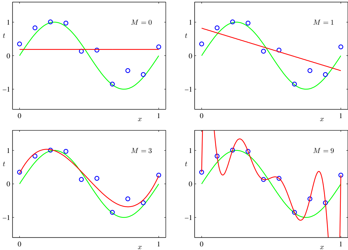
图 1.4: 不同阶数的多项式曲线，用红色曲线表示，拟合了图1.2中的数据集。
