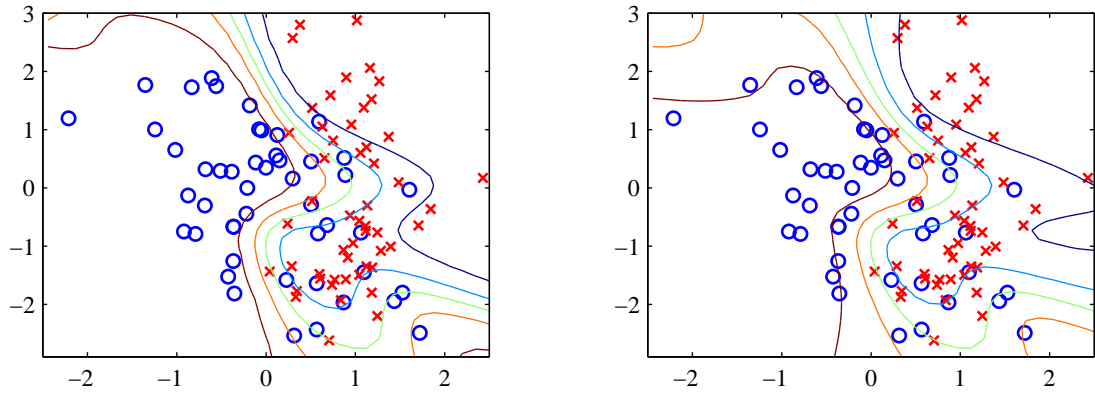
图 5.23: 对于一个具有8个隐含结点带有tanh激活函数和一个logistic sigmoid输出结点的贝叶斯网络应用拉普拉斯近似的说明。权参数使用缩放的共轭梯度方法得到, 超参数 \alpha 使用模型证据框架确定。左图是使用基于参数的 w_{MAP} 的点估计的简单近似 (5.185) 得到的结果, 其中绿色曲线表示 y = 0.5 的决策边界, 其他的轮廓线对应于 y = 0.1, 0.3, 0.7 和 0.9 的输出概率。右图是使用公式 (5.190) 得到的对应的结果。注意, 求边缘概率分布的效果是扩散了轮廓线, 使得预测的置信度变低, 从而在每个输入点 x 处, 后验概率分布向着0.5的方向偏移, 而 y = 0.5 的边界本身不受影响。
