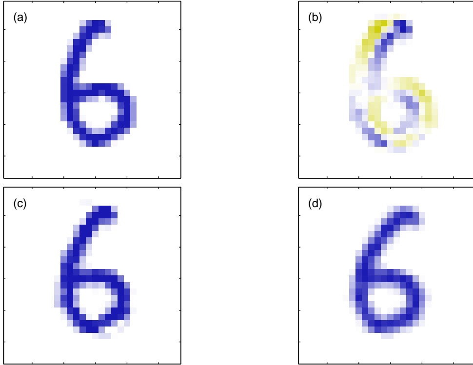
图 5.16: (a)原始的手写数字 \boldsymbol{x} , (b)对应于无穷小顺时针旋转的切向量 \boldsymbol{\tau} , 其中蓝色和黄色分别对应于正值和负值, (c)将来自这个切向量的微小贡献作用于原始图像的结果, 得到了 \boldsymbol{x} + \epsilon\boldsymbol{\tau} , 其中 \epsilon = 15 度。(d)真实的图像旋转, 用作对比。
