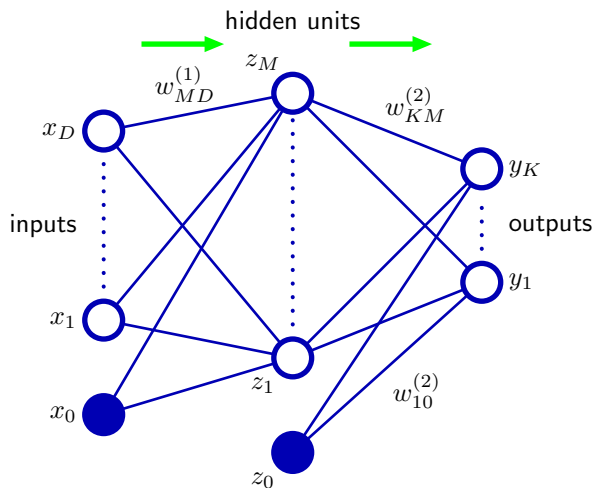
图 5.1: 对应于公式 (5.7) 的两层神经网络的网络图。输入变量、隐含变量、输出变量都表示为结点, 权重参数被表示为结点之间的链接, 其中偏置参数被表示为来自额外的输入变量 x_0 和隐含变量 z_0 的链接。箭头表示信息流在网络中进行前向传播的方向。
