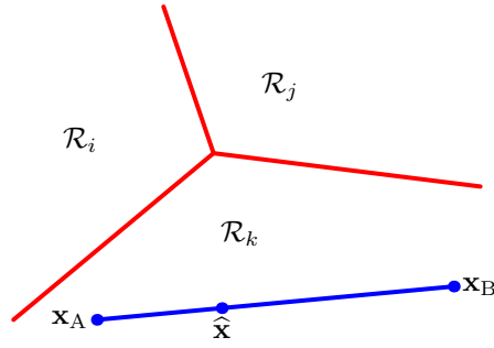
图 4.3: 多类判别函数的决策区域的说明, 决策边界用红色表示。如果两个点 \mathbf{x}_A 和 \mathbf{x}_B 位于同一个决策区域 \mathcal{R}_k , 那么任何位于连接这两个点的线段上的点 \hat{\mathbf{x}} 一定位于区域 \mathcal{R}_k 内, 因此决策区域一定是单连通的、凸的。
