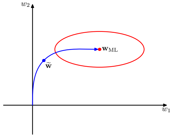
图 5.13: 在二次误差函数的情况下, 关于早停止可以给出与权值衰减类似的结果的原因说明。椭圆给出了常数误差函数的轮廓线, w_{ML} 表示误差函数的最小值。如果权向量的起始点为原点, 按照局部负梯度的方向移动, 那么它会沿着曲线给出的路径移动。通过对训练过程早停止, 我们找到了一个权值向量 \tilde{w} 。定性地说, 它类似于使用简单的权值衰减正则化项, 然后最小化正则化误差函数的方法得到的权值。通过与图 3.15 进行对比, 我们可以看到这一点。
