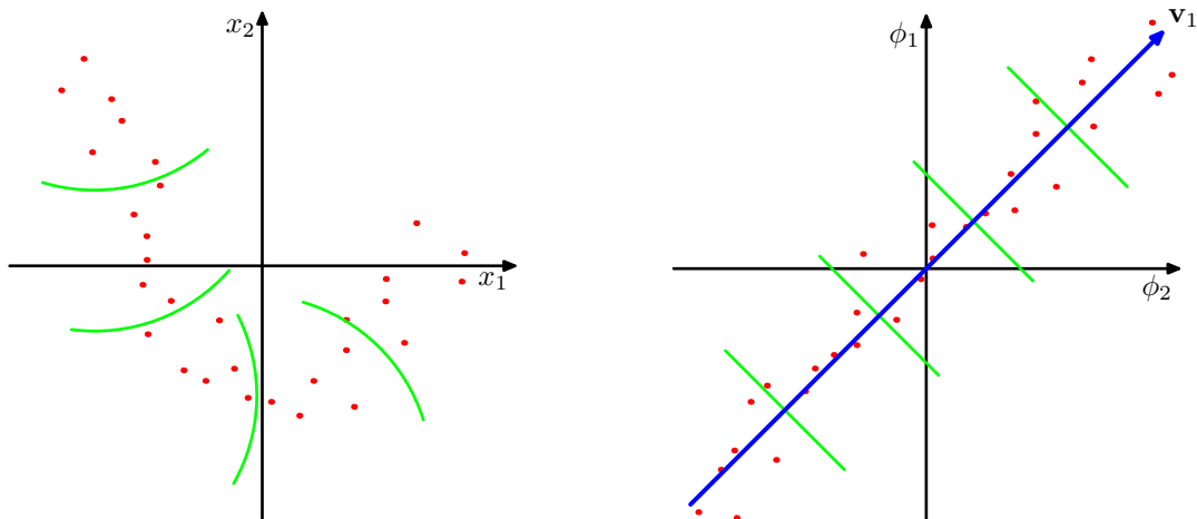
图 12.16: 核PCA的图形化说明。原始数据空间中的数据集（左图）被非线性变换 \phi(\mathbf{x}) 投影到特征空间中（右图）。通过在特征空间中执行PCA，我们得到了主成分，其中第一主成分用蓝色表示，记作向量 \mathbf{v}_1 。特征空间中的绿色直线表示特征空间中在第一主成分上的线性投影，它对应于原始数据空间中的非线性投影。注意，通常不可能在 \mathbf{x} 空间中表示非线性主成分。
