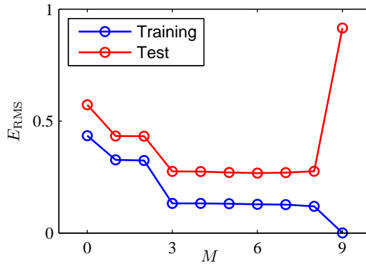
图 1.5: 公式 (1.3) 定义的根均方误差的图像, 分别在训练数据集上和独立的测试数据集上对于不同的 M 进行了计算。
