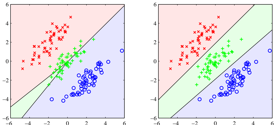
图 4.5: 由三个类别组成的人工数据集的例子, 训练数据点分别用红色 (×)、绿色 (+)、蓝色 (○) 标出。直线表示决策边界, 背景颜色表示决策区域代表的类别。左图是一个使用最小平方判别函数的结果。我们看到分配到绿色类别的输入空间的区域过小, 大部分来自这个类别的点都被错误分类。右图是使用 4.3.2 节描述的使用 logistic 回归的结果, 给出了训练数据的正确分类情况。
