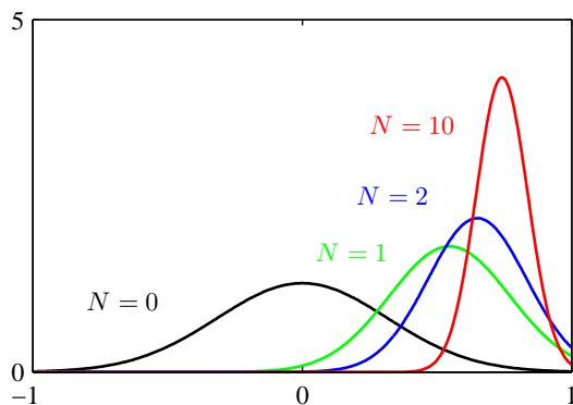
图 2.12: 高斯分布的均值 \mu 的贝叶斯推断, 其中我们假设方差已知。曲线展示了 \mu 上的先验概率分布 (标记为 N = 0 的曲线), 在这种情况下, 它本身是一个高斯分布。同时给出的还有随着数据点数量 N 的增大, 公式 (2.140) 给出的后验概率分布。数据点由均值为0.8、方差为0.1的高斯分布生成, 先验分布的均值被选择为0。在先验概率分布和似然函数中, 方差都被设置为了真实值。
