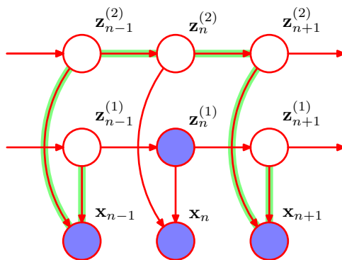
图 13.20: 绿色标记的路径在观测结点 x_{n-1} 和 x_{n+1} 处是头到头的, 在非观测结点 z_{n-1}^{(2)} , z_n^{(2)} 和 z_{n+1}^{(2)} 处是头到尾的。因此路径没有被阻隔, 从而条件独立性质 (13.5) 对于因子HMM模型各个潜在链不成立。结果, 这个模型没有高效的精确E步骤。
