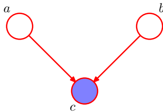
图 8.20: 与图 8.19 相同，但是以结点 c 的值为条件。这张图中，引入条件结点使得 a 和 b 之间产生了依赖关系。
