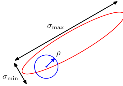
图 11.10: 使用Metropolis-Hastings算法, 用一个各项同性的高斯提议分布 (蓝色圆圈) 从一个具有相关性的多元高斯分布 (红色椭圆) 中采样, 这个多元高斯分布在不同的方向上的标准差的数值相当不同。为了让拒绝率较低, 提议分布的标度 \rho 应该与最小的标准差 \sigma_{\min} 处于同一个量级, 这会产生随机游走的行为, 达到独立的状态所需的步骤数的量级为 (\sigma_{\max}/\sigma_{\min})^2 , 其中 \sigma_{\max} 是最大的标准差。
