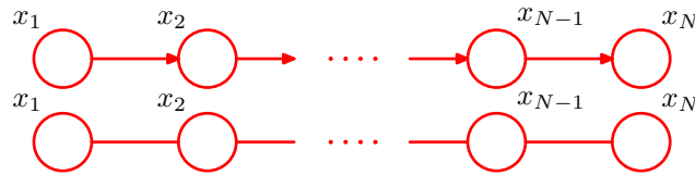
图 8.32: (a) 有向图的例子。 (b) 等价的无向图。
