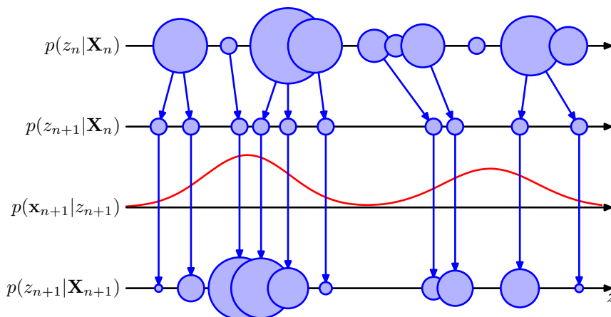
图 13.23: 对于一维潜在空间, 粒子滤波操作的图形表示。在时刻 n , 后验概率分布 p(z_n | \mathbf{X}_n) 被表示为混合概率分布, 用圆圈表示, 它的大小正比于权值 w_n^{(l)} 。之后, 一组 L 个样本从这个概率分布中抽取, 新的权值 w_{n+1}^{(l)} 使用 p(\mathbf{x}_{n+1} | z_{n+1}^{(l)}) 计算。
