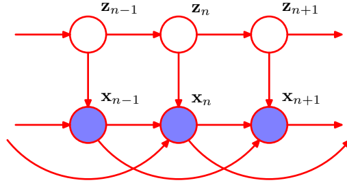
图 13.17: 自回归隐马尔可夫模型的一部分, 其中, 观测 x_n 的概率分布依赖于之前的观测的子集以及隐状态 z_n 。在这个例子中, x_n 的分布依赖于两个之前的观测 x_{n-1} 和 x_{n-2} 。
