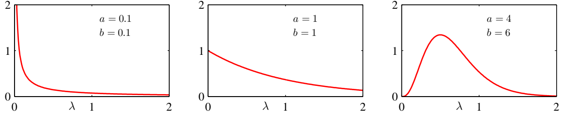
图 2.13: 对于不同的参数 a 和 b , 公式 (2.146) 定义的Gamma分布 \text{Gam}(\lambda | a, b) 的图像。
