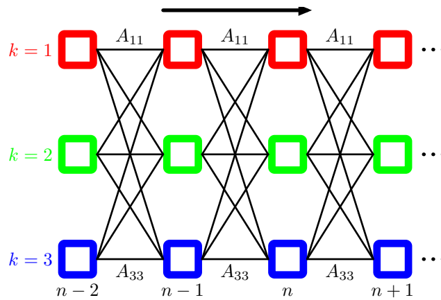
图 13.7: 如果我们将图13.6所示的状态转移图在时间上展开, 那么我们就得到了潜在状态的晶格图表示或者格子图表示。图的每一列对应于一个潜在变量 z_n 。
