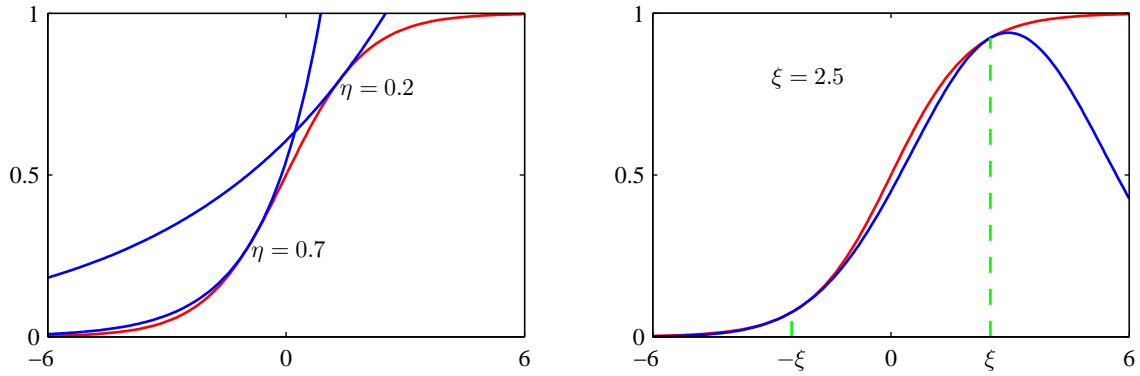
图 10.12: 左图中, 红色曲线给出了公式 (10.134) 定义的 logistic sigmoid 函数 \sigma(x) 。同时给出的还有两个指数上界 (10.137) 的例子, 用蓝色曲线表示。右图再次用红色曲线给出了 logistic sigmoid 函数。同时给出的还有高斯下界 (10.144), 用蓝色曲线表示。这里, 参数 \xi = 2.5 , 界限在 x = \xi 和 x = -\xi 出事精确的, 用绿色曲线标记。
