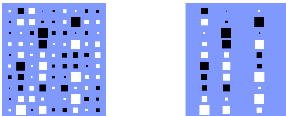
图 12.14: 矩阵 \mathbf{W} 的 Hinton 图, 其中矩阵的每个元素被表示为一个正方形, 白色表示正值, 黑色表示负值, 正方形的面积正比于那个元素的大小。人工生成的数据集由 300 个数据点构成, 数据点从一个 D = 10 维的高斯分布中采样, 高斯分布在 3 个方向上的标准差为 1.0, 在剩余的 7 个方向上的标准差为 0.5。数据空间的维度为 D = 10 , 在 M = 3 个方向上的方差大于剩余的 7 个方向上的方差。左图给出了使用最大似然方法的概率 PCA 的结果, 右图给出了贝叶斯 PCA 的对应的结果。我们看到通过压制 6 个多余的自由度的方式来发现维度的合适的值。
