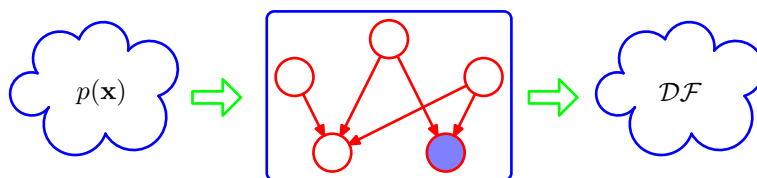
图 8.25: 我们可以将图模型 (在这幅图中是有向图) 看成滤波器。当且仅当概率分布 p(\mathbf{x}) 满足有向分解性质 (8.5) 时, p(\mathbf{x}) 才可以通过滤波器。通过滤波器的所有可能的概率分布 p(\mathbf{x}) 被记作 \mathcal{DF} 。我们也可以根据概率分布是否满足由图的 d -划分性质表示的所有的条件独立性质来使用图对概率分布进行过滤。 d -划分定理表明, 这两种滤波方式得到的概率分布集合 \mathcal{DF} 是相同的。
