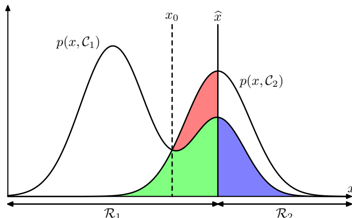
图 1.24: 两个类别的联合概率分布 p(x, C_k) 与 x 的关系, 以及决策边界 x = \hat{x} 。 x \geq \hat{x} 的值被分类为 C_2 , 因此属于决策区域 \mathcal{R}_2 , 而 x < \hat{x} 的值被分类为 C_1 , 属于区域 \mathcal{R}_1 。错误出现在蓝色、绿色和红色区域, 从而对于 x < \hat{x} , 错误的来源是将属于类别 C_2 的点错分到类别 C_1 (表示为红色区域与绿色区域的总和), 相反对于 x \geq \hat{x} 的点, 错误的来源是将属于类别 C_1 的点错分到类别 C_2 (表示为蓝色区域)。当我们改变决策区域的位置 \hat{x} 时, 绿色区域和蓝色区域的总面积是一个常数, 而红色区域的面积发生改变。 \hat{x} 的最优选择是 p(x, C_1) 的曲线与 p(x, C_2) 的曲线相交, 对应于 \hat{x} = x_0 , 因为此时红色区域消失。这等价于最小化错误分类率的决策规则, 这个规则将 x 分配到具有最大的后验概率 p(C_k | x) 的区域中。
