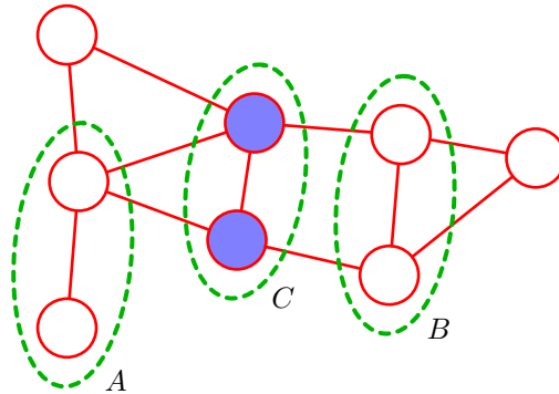
图 8.27: 无向图的一个例子，其中从集合 A 中的任意结点到集合 B 中的任意结点的每条路径都通过集合 C 中的至少一个结点。结果，对于所有由这个图描述的任意概率分布，以 C 为条件， A 与 B 都条件独立。
