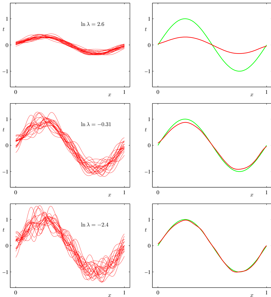
图 3.5: 模型复杂度对于偏置和方差的依赖的说明。模型的复杂度由正则化参数 \lambda 控制, 数据集是第1章中的正弦数据。有 L = 100 个数据集, 每个数据集有 N = 25 个数据点, 每个模型有24个高斯基函数, 从而参数的总数为 M = 25 (包括偏置参数)。左侧一列给出了对于不同的 \ln \lambda 值, 根据数据集拟合模型的结果。为了清晰起见, 我们只给出了100个拟合模型中的20个。右侧一列给出了对应的100个拟合的均值 (红色) 以及用于生成数据集的正弦函数 (绿色)。
