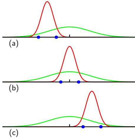
图 1.15: 这幅图说明了使用最大似然方法确定高斯分布的方差时, 偏移是如何产生的。绿色曲线表示真实的高斯分布, 数据点是根据这个概率分布生成的。三条红色曲线表示对三个数据集拟合得到的高斯概率分布, 每个数据集包含两个蓝色的数据点, 使用公式 (1.55) 和公式 (1.56) 给出的最大似然的结果进行拟合。对三个数据集求平均, 均值是正确的, 但是方差被系统地低估了, 因为它是相对样本均值进行测量的, 而不是相对真实的均值进行测量。
