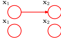
图 8.9: (a)全连接的图描述了两个 K 状态离散变量上的一般的分布, 具有 K^2 - 1 给参数。(b)通过丢弃结点之间的链接, 参数的数量减小到了 2(K - 1) 。
