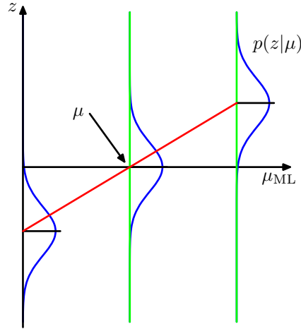
图 2.11: 在高斯分布的情形中, 图 2.10 所示的回归函数的形式是一条直线, 用红色标记出, 其中 \theta 对应于 \mu_{ML} 。在这种情况下, 随机变量 z 对应于对数似然函数的导数, 由 -(x - \mu_{ML})/\sigma^2 给出, 定义了回归函数的期望是一条直线, 由 -(\mu - \mu_{ML})/\sigma^2 给出。回归函数的根对应于真实的均值 \mu 。
