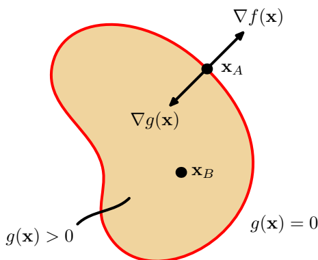
图 E.3: 满足不等式限制条件 g(\mathbf{x}) \geq 0 下, 最大化 f(\mathbf{x}) 的问题的例子。
