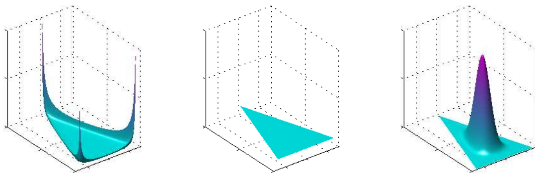
图 2.5: 三个变量上的狄利克雷分布的图像, 其中两个水平轴是单纯形平面上的坐标轴, 垂直轴对应于概率密度的值。这里 \{\alpha_k\} = 0.1 对应于左图, \{\alpha_k\} = 1 对应于中图, \{\alpha_k\} = 10 对应于右图。
