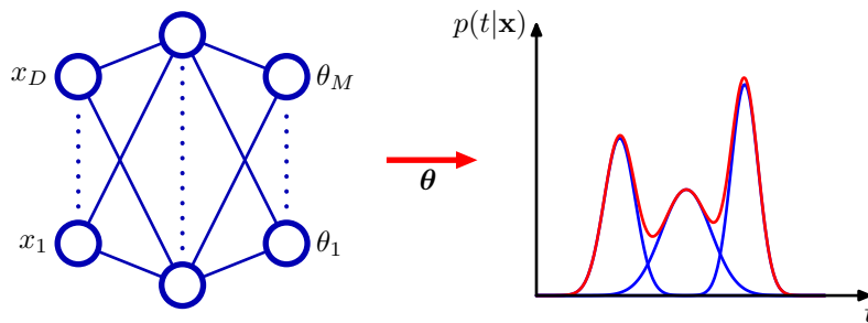
图 5.20: 混合密度网络 (mixture density network) 可以表示一般的条件概率密度 p(t | \mathbf{x}) ，方法为：考虑 t 的一个参数化的混合模型，它的参数由以 \mathbf{x} 为输入的神经网络的输出确定。
