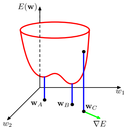
图 5.5: 误差函数 E(\mathbf{w}) 的几何表示。其中, 误差函数被表示为权空间上的一个曲面。点 \mathbf{w}_A 是一个局部最小值, 点 \mathbf{w}_B 是全局最小值。在任意点 \mathbf{w}_C 处, 误差函数的局部梯度由向量 \nabla E 给出。
