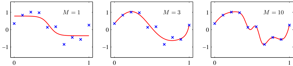
图 5.9: 使用从正弦数据集中抽取的10个数据点训练的两层神经网络的例子。各图分别给出了使用 M = 1, 3, 10 个隐含单元调节网络的结果，调节的方法是使用放缩的共轭梯度算法来最小化平方和误差函数。
