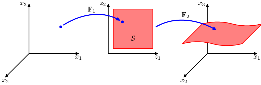
图 12.20: 图12.19的网络表示的映射的集合表示, 其中输入单元的数量为 D = 3 , 中间隐含层单元的数量为 M = 2 。函数 F_2 表示从 M 维空间 S 到 D 维空间的一个映射, 因此定义了空间 S 嵌入到原始 x 空间的方式。由于映射 F_2 可以是非线性的, 因此 S 嵌入的空间可以不是平面, 如图所示。这样, 映射 F_1 定义了原始 D 维空间中的一个点到 M 维子空间 S 中的投影。
