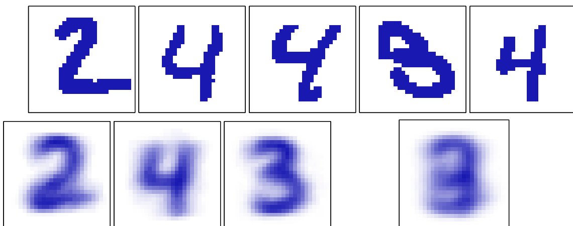
图 9.10: 伯努利混合模型的例子。上面一行给出了将手写数字数据集从灰度图转化为二值图之后的例子，转化时使用的阈值为0.5。下面一行中，最开始的三张图像展示了混合模型三个分量的参数 \mu_{ki} 。作为对比，我们也使用一个单一的多元伯努利分布对同样的数据进行了拟合，同样使用了最大似然方法。这对应于将每个像素点求平均，结果如下面一行最右侧的图所示。
