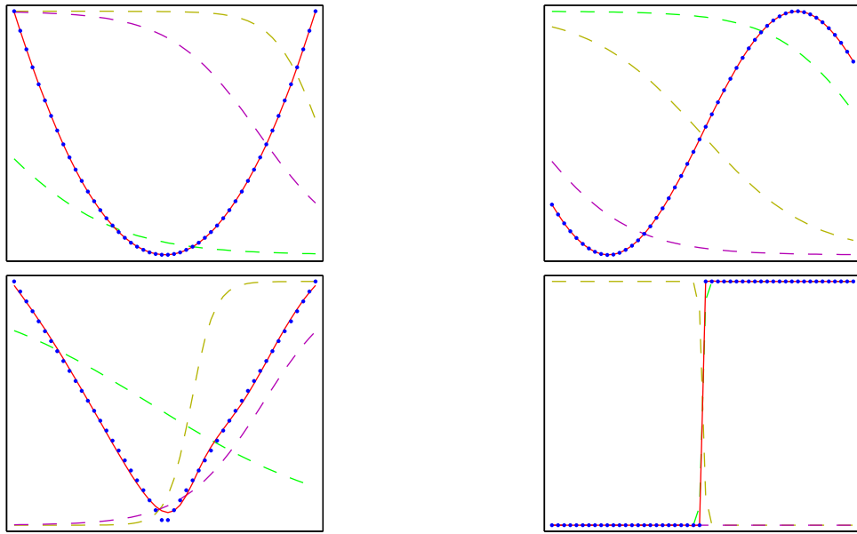
图 5.3: 多层感知器的能力说明, 它用来近似四个不同的函数。(a) f(x) = x^2 , (b) f(x) = \sin(x) , (c) f(x) = |x| , (d) f(x) = H(x) , 其中 H(x) 是一个硬阶梯函数。在每种情况下, N = 50 个数据点 (用蓝点表示) 从区间 (-1, 1) 中均匀分布的 x 中进行取样, 然后计算出对应的 f(x) 值。这些数据点之后用来训练一个具有 3 个隐含单元的两层神经网络, 隐含单元的激活函数为 \tanh 函数, 输出为线性输出单元。生成的网络函数使用红色曲线表示, 三个隐含单元的输出用三条虚线表示。
