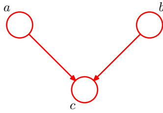
图 8.19: 3 结点图三个例子中的最后一个例子，这些例子用来研究图模型中的条件独立性质。这张图与前两个例子的性质相当不同。
