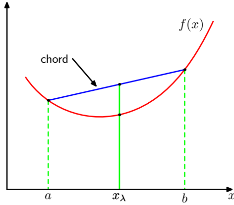
图 1.31: 凸函数 f(x) 的每条弦（蓝色表示）位于函数上或函数上方，函数用红色曲线表示。
