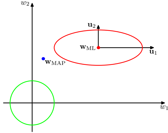
图 3.15: 似然函数的轮廓线 (红色) 和先验概率分布 (绿色), 其中参数空间中的坐标轴被旋转, 与 Hessian 矩阵的特征向量 \mathbf{u}_i 对齐。对于 \alpha = 0 , 后验概率分布的众数由最大似然解 \mathbf{w}_{ML} 给出, 而对于非零的 \alpha , 众数位于 \mathbf{w}_{MAP} = \mathbf{m}_N 的位置。在方向 w_1 上, 由公式 (3.87) 定义的特征值 \lambda_1 与 \alpha 相比较小, 因此 \lambda_1/(\lambda_1 + \alpha) 接近零, 对应的 w_1 的 MAP 值也接近零。相反, 在 w_2 的方向上, 特征值 \lambda_2 与 \alpha 相比较较大, 因此 \lambda_2/(\lambda_2 + \alpha) 接近 1, w_2 的 MAP 值接近于最大似然值。
