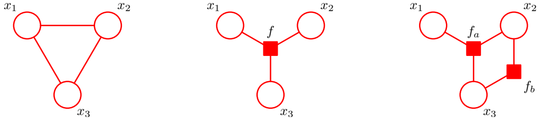
图 8.41: (a) 一个无向图, 有一个单一的团块势函数 \psi(x_1, x_2, x_3) 。 (b) 一个因子图, 因子 f(x_1, x_2, x_3) = \psi(x_1, x_2, x_3) , 它表示与无向图相同的概率分布。 (c) 一个不同的因子图, 表示相同的概率分布, 它的因子满足 f_a(x_1, x_2, x_3)f_b(x_2, x_3) = \psi(x_1, x_2, x_3) 。
