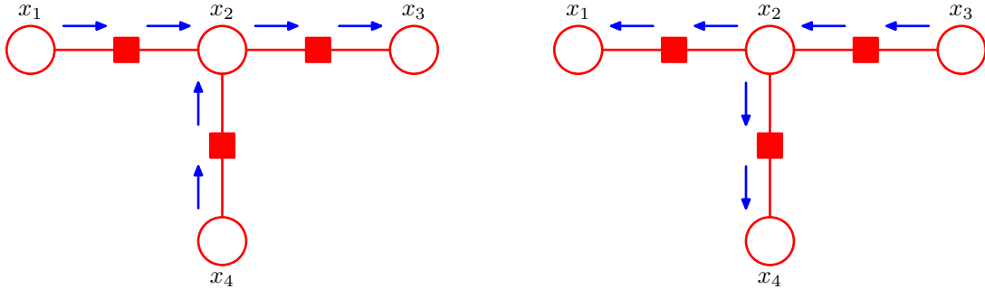
图 8.52: 应用于图8.51给出的图的加和-乘积算法的信息流。(a)从叶结点 x_1 和 x_4 向根结点 x_3 传递。(b)从根结点向叶结点传递。
