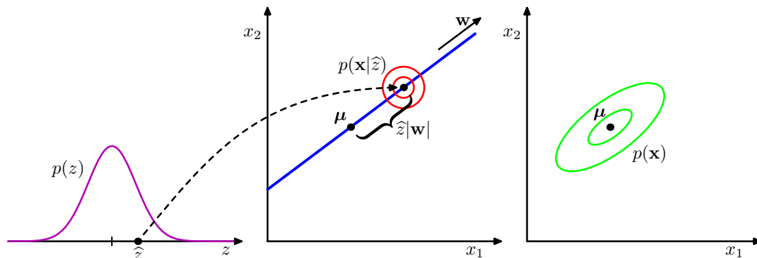
图 12.9: 概率PCA模型的生成式观点的说明, 数据空间为二维, 潜在空间为一维。一个观测数据点 \mathbf{x} 的生成方式为: 首先从潜在变量的先验分布 p(z) 中抽取一个潜在变量的值 \hat{z} , 然后从一个各向同性的高斯分布(用红色圆圈表示)中抽取一个 \mathbf{x} 的值, 这个各向同性的高斯分布的均值为 \mathbf{w}\hat{z} + \boldsymbol{\mu} , 协方差为 \sigma^2\mathbf{I} 。绿色椭圆画出了边缘概率分布 p(\mathbf{x}) 的密度轮廓线。
