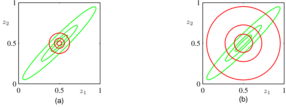
图 10.2: 两种形式的KL散度的对比。绿色轮廓线对应于两个变量 z_1 和 z_2 上的相关高斯分布 p(\mathbf{z}) 的1、2、3个标准差的位置，红色轮廓线表示相同变量上的近似分布 q(\mathbf{z}) 的同样位置。近似分布 q(\mathbf{z}) 由两个独立的一元高斯分布的乘积给出，(a)图中，参数通过最小化Kullback-Leibler散度 \text{KL}(q \parallel p) 的方式获得，(b)图中，参数通过最小化相反的Kullback-Leibler散度 \text{KL}(p \parallel q) 的方式获得。
