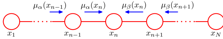
图 8.38: 对于结点链上的一个结点 x_n , 边缘概率分布可以通过下面的方式求得: 将两个信息 \mu_\alpha(x_n) 和 \mu_\beta(x_n) 相乘, 然后归一化。这些信息本身可以通过从结点链的两侧向结点 x_n 传递信息的方式递归地计算。
