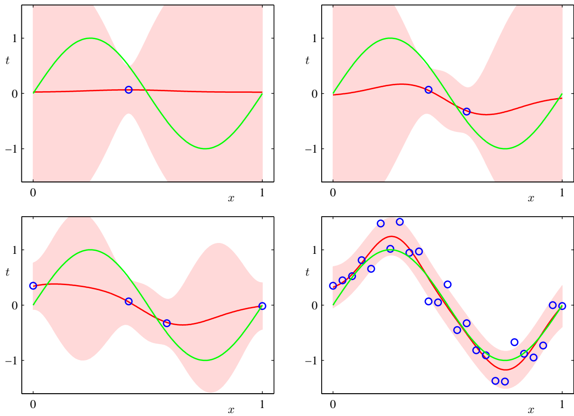
图 3.8: 包含9个高斯基函数 (3.4) 的模型的预测分布 (3.58), 使用了1.1节的人工生成的正弦数据集。详细的讨论见正文。
