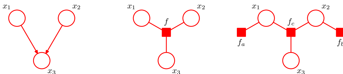
图 8.42: (a) 一个有向图，可以分解为 p(x_1)p(x_2)p(x_3 | x_1, x_2) 。(b) 一个因子图，表示与有向图相同的概率分布，它的因子满足 f(x_1, x_2, x_3) = p(x_1)p(x_2)p(x_3 | x_1, x_2) 。(c) 一个不同的因子图，表示同样的概率分布，因子为 f_a(x_1) = p(x_1) , f_b(x_2) = p(x_2) , f_c(x_1, x_2, x_3) = p(x_3 | x_1, x_2) 。
