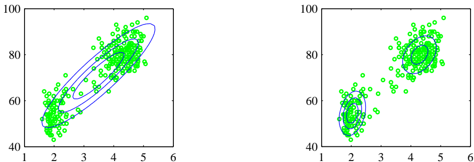
图 2.21: 老忠实间歇喷泉数据点, 其中蓝色曲线给出了常数概率密度的轮廓线。左图是一个单一的高斯概率分布, 已经使用最大似然法根据数据进行了调参。注意, 这个概率分布未能描述数据中的两个聚集区域, 并且把大部分的概率质量放在了中心区域, 而这个区域的数据相对稀疏。右图是两个高斯概率分布进行线性组合得到的概率分布, 已经使用第9章将要介绍的方法使用最大似然的方式根据数据进行了调参, 它给出了关于数据的一个更好的表示。
