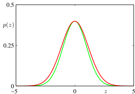
图 11.7: 从高斯分布 p(z) (绿色曲线) 中进行拒绝采样的例子, 提议分布 q(z) 也是一个高斯分布, 它的缩放版本 kq(z) 用红色曲线表示。
