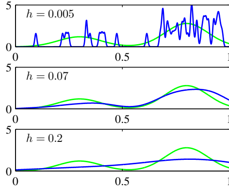
图 2.25: 公式 (2.250) 给出的核密度模型的例子。数据集与图2.24中用于说明直方图方法时使用的数据集相同。我们看到, h 的作用相当于平滑参数, 如果它被设置得过小(最上方的图), 结果是一个噪声非常大的概率模型, 而如果它被设置得过大(最下方的图), 那么用于生成数据的概率分布(绿色曲线表示)的双峰性质被抹去了。 h 取某个中等大小的值时, 可以得到最好的密度模型(中间的图)。
