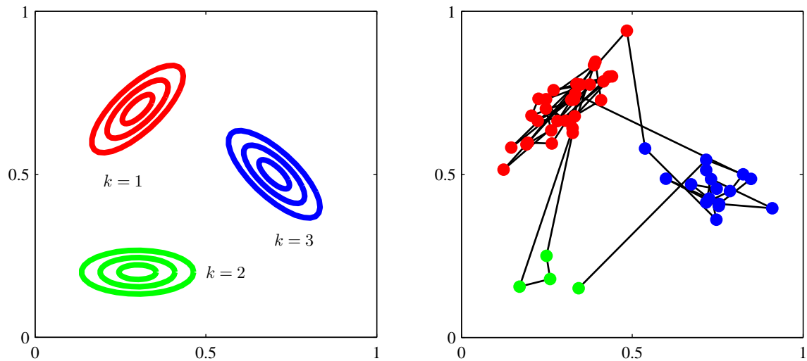
图 13.8: 从一个隐马尔科夫模型中进行采样的例子, 这个模型的潜在变量 z 有三个状态, 发射概率 p(\mathbf{x} | z) 是高斯概率, 其中 \mathbf{x} 是二维的。(a)发射概率密度为常数的轮廓线, 对应于潜在变量的三个状态。(b)从隐马尔科夫模型中抽取的50个样本点, 数据点的颜色对应于生成它们的分量的颜色, 数据点之间的连线表示连续的观测。这里, 转移矩阵是固定的。在任何状态, 都有5%的概率转移到每个其他的状态, 有90%的概率保持相同的状态。
