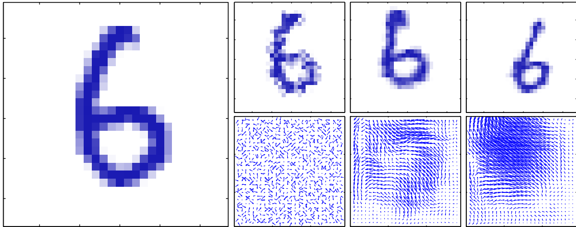
图 5.14: 对手写数字进行人工形变的说明。原始图像见左图。在右图中, 上面一行给出了三个经过了形变的数字, 对应的位移场在下面一行给出。这些位移场按照下面的方法生成: 在每个像素处, 对唯一 \Delta x, \Delta y \in (0, 1) 进行随机取样, 然后分别与宽度为 0.01, 30, 60 的高斯分布做卷积, 进行平滑。
