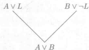
图 15.3 归结原理例示
