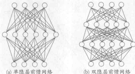
图 5.6 多层前馈神经网络结构示意图
