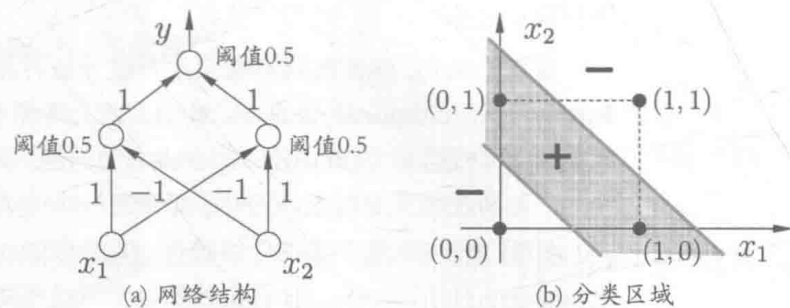
图 5.5 能解决异或问题的两层感知机
