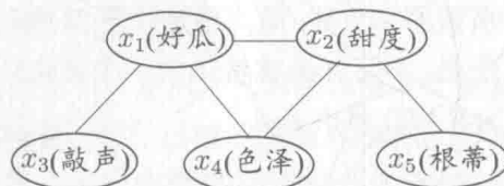
图 7.4 图 7.2 对应的道德图
