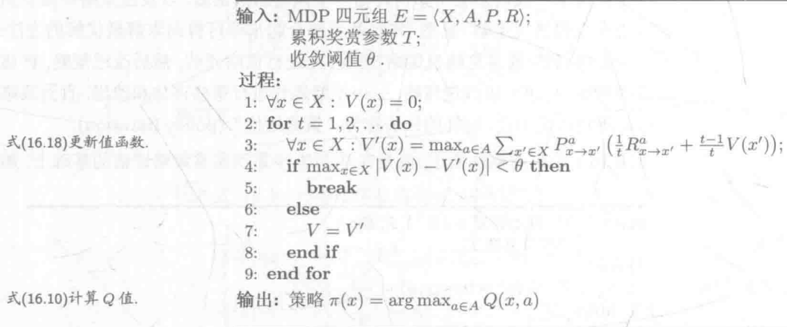
图 16.9 基于 T 步累积奖赏的值迭代算法
