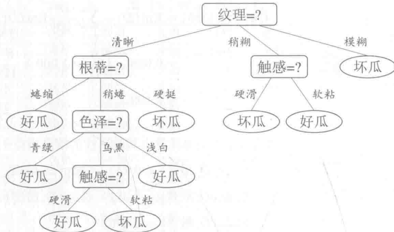
图 4.4 在西瓜数据集 2.0 上基于信息增益生成的决策树
