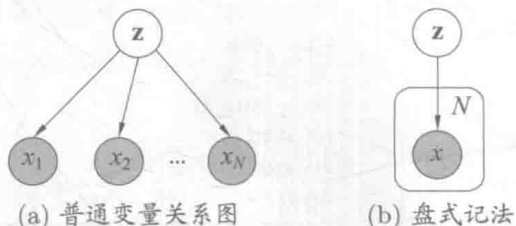
图 14.10 盘式记法的例示
