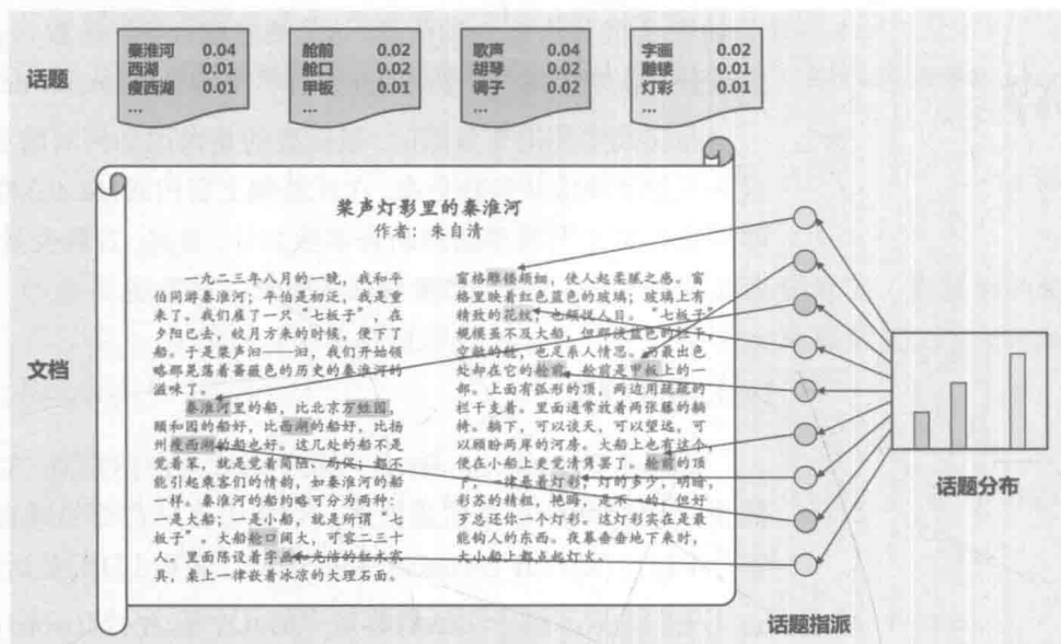
图 14.11 LDA 的文档生成过程示意图
