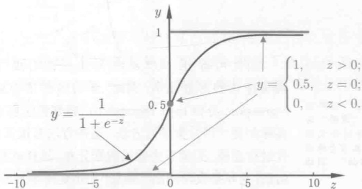
图 3.2 单位阶跃函数与对数几率函数
