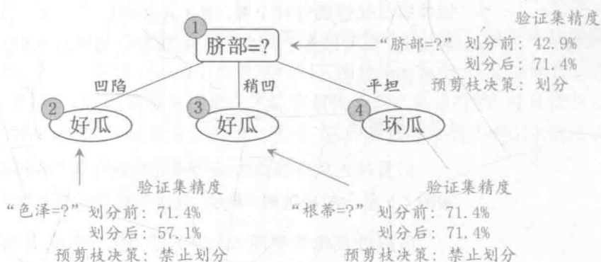
图 4.6 基于表 4.2 生成的预剪枝决策树
