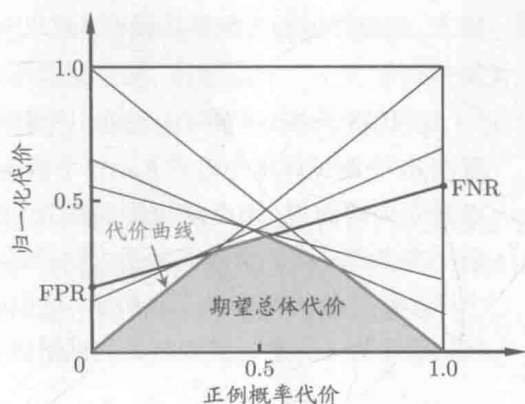
图 2.5 代价曲线与期望总体代价
