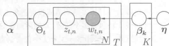
图 14.12 LDA 的盘式记法图
