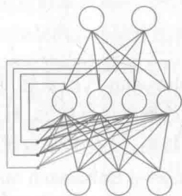
图 5.13 Elman 网络结构
