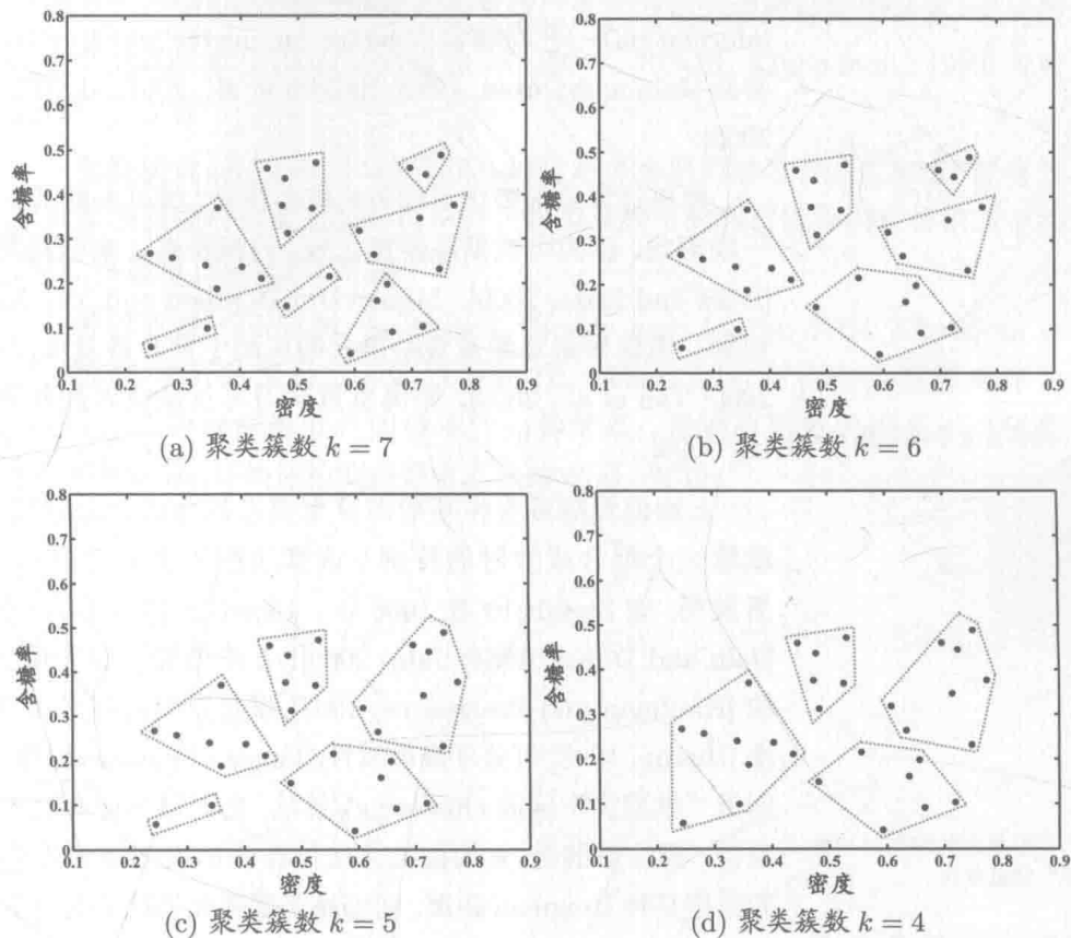
图 9.13 西瓜数据集 4.0 上 AGNES 算法(采用 d_{\max} )在不同聚类簇数( k = 7, 6, 5, 4 )时的簇划分结果. 样本点用“●”表示, 红色虚线显示出簇划分.
