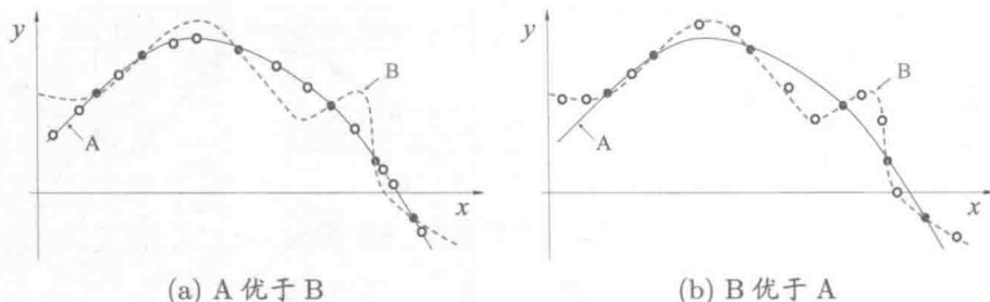
图 1.4 没有免费的午餐. (黑点: 训练样本; 白点: 测试样本)
