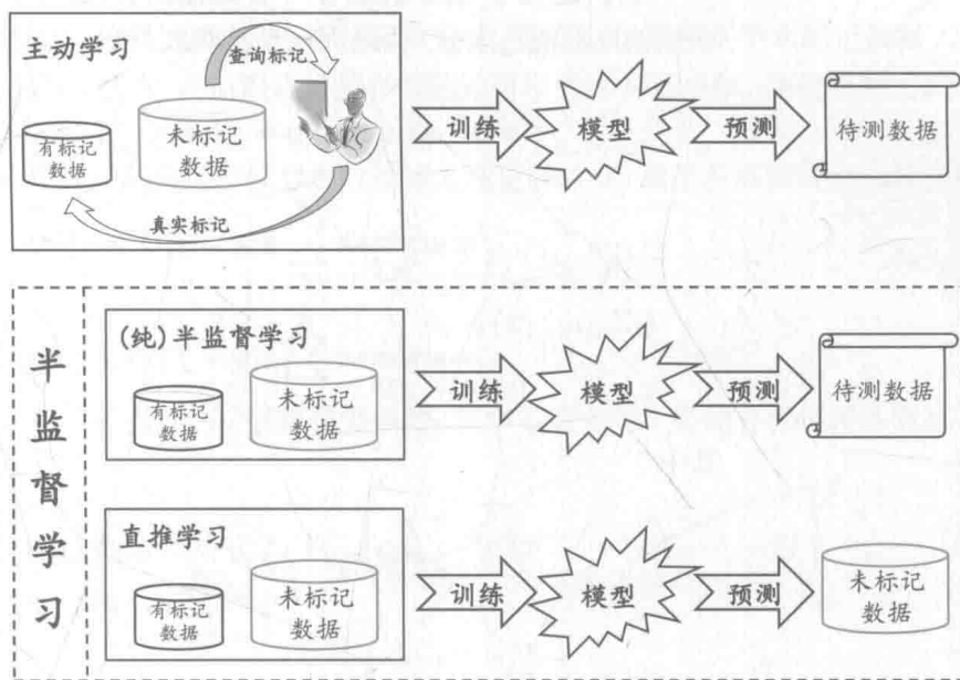
图 13.2 主动学习、(纯)半监督学习、直推学习
