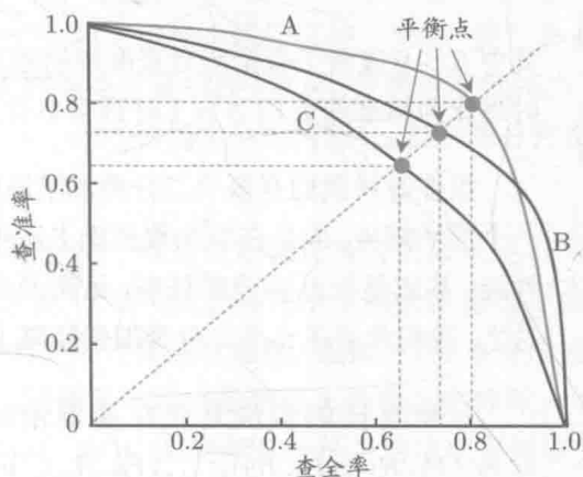
图 2.3 P-R曲线与平衡点示意图
