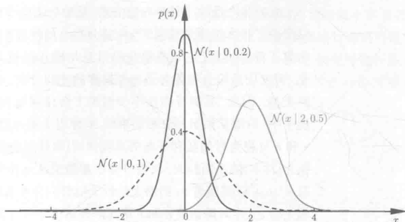
附图C.3 高斯分布的概率密度函数
