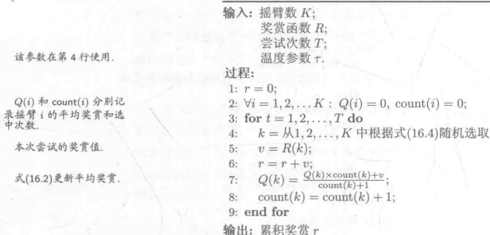
图 16.5 Softmax 算法
