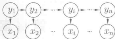
图 14.1 隐马尔可夫模型的图结构
