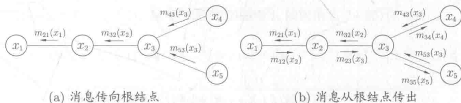
图 14.8 信念传播算法图示
