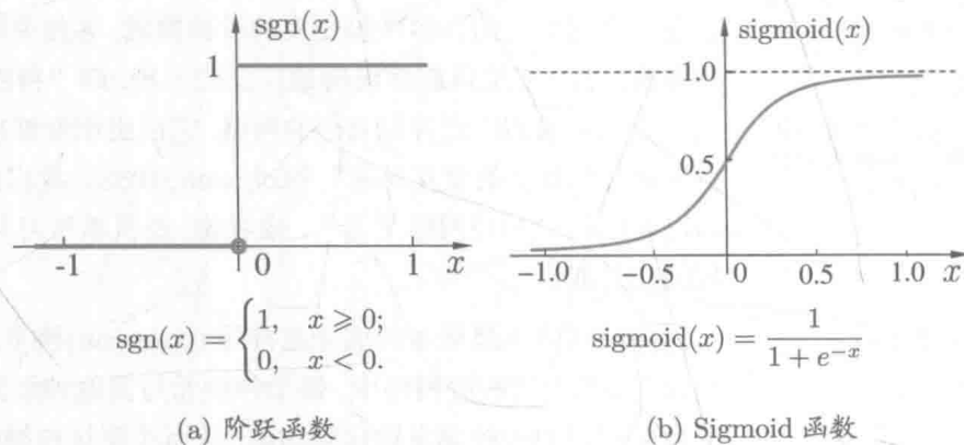
图 5.2 典型的神经元激活函数
