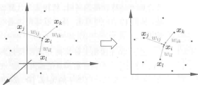
图 10.9 高维空间中的样本重构关系在低维空间中得以保持
