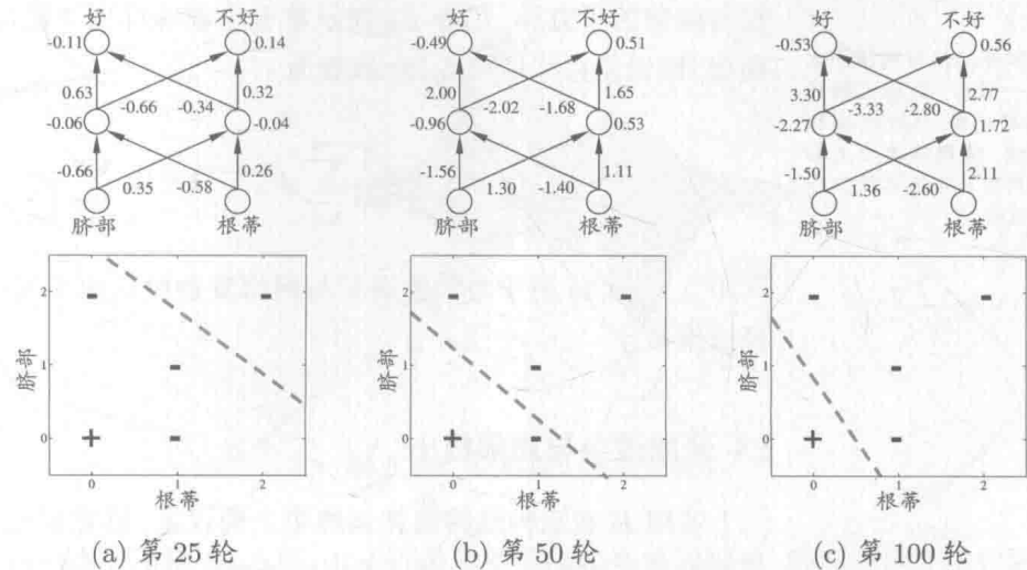
图 5.9 在2个属性、5个样本的水瓜数据上, BP网络参数更新和分类边界的变化情况
