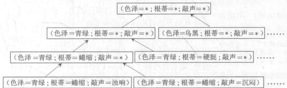
图 1.1 西瓜问题的假设空间
