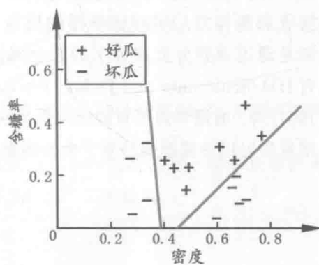
图 4.14 图 4.13 多变量决策树对应的分类边界
