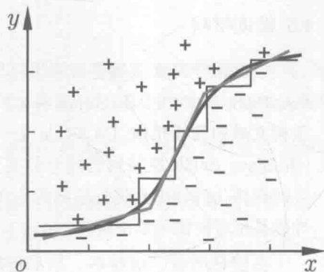
图 4.12 决策树对复杂分类边界的分段近似
