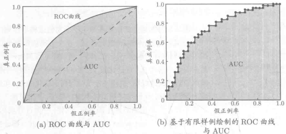
图 2.4 ROC 曲线与 AUC 示意图
