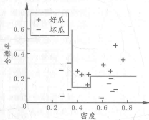
图 4.11 图 4.10 决策树对应的分类边界
