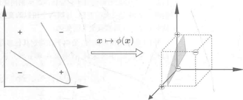
图 6.3 异或问题与非线性映射
