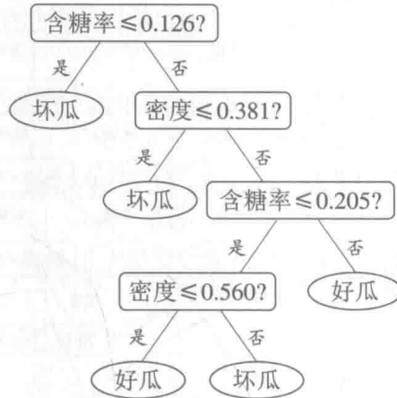
图 4.10 在西瓜数据集 3.0α 上生成的决策树
