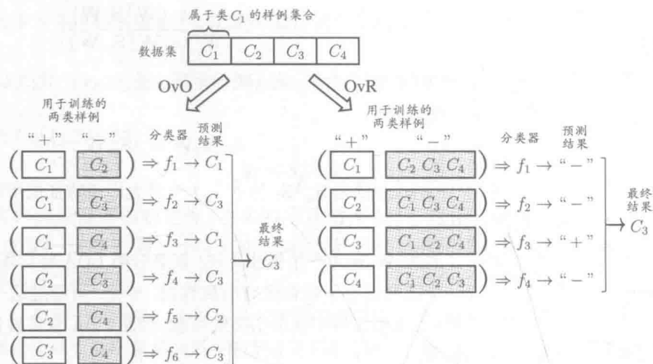
图 3.4 OvO 与 OvR 示意图
