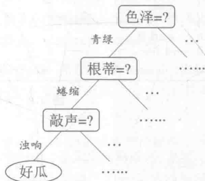
图 4.1 西瓜问题的一棵决策树
