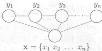
图 14.6 链式条件随机场的图结构
