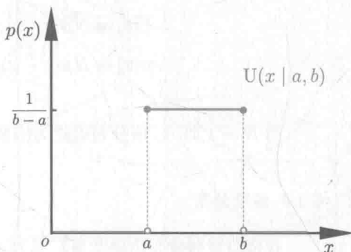
附图C.1 均匀分布的概率密度函数
