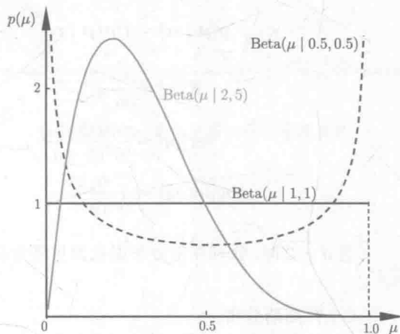
附图C.2 贝塔分布的概率密度函数
