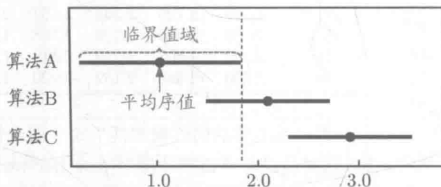
图 2.8 Friedman 检验图
