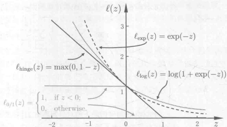
图 6.5 三种常见的替代损失函数: hinge损失、指数损失、对率损失
