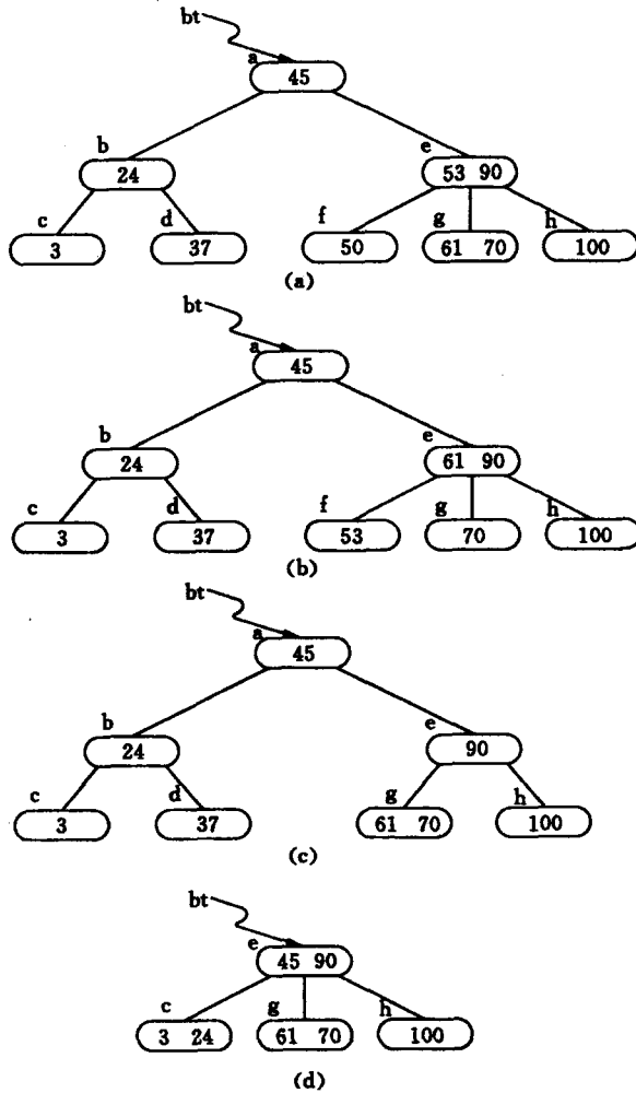
图 9.17 在 B-树中删除关键字的情形
