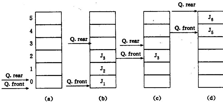
图 3.12 头、尾指针和队列中元素之间的关系
