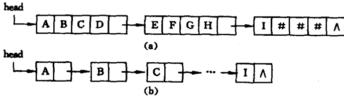
图 4.2 串值的链表存储方式 (a) 结点大小为 4 的链表; (b) 结点大小为 1 的链表
