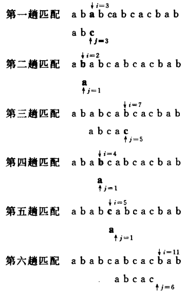
图 4.3 算法 4.5 的匹配过程
