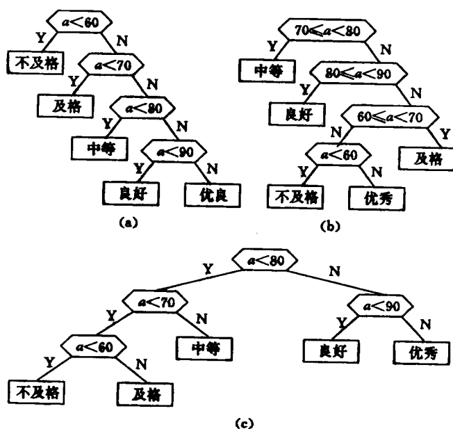
图 6.23 转换五级分制的判定过程
