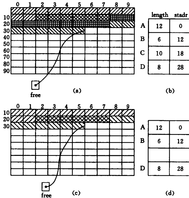
图 8.12 堆存储管理示意图
