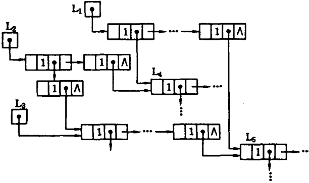
图 8.9 含有共享子表的广义表
