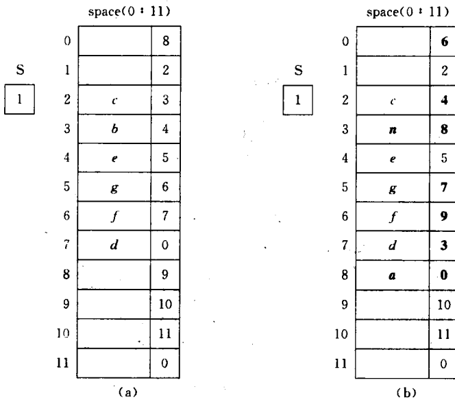
图 2.11 运算前后的静态链表
