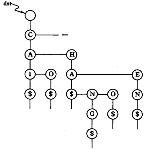
图 9.20 双链树示例
