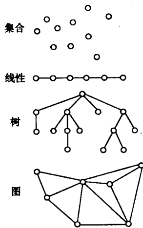
图 1.5 4 类基本结构关系图
