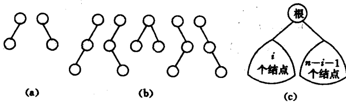
图 6.30 二叉树的形态
