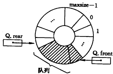
图 3.13 循环队列示意图
