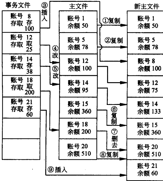
图 12.4 银行账目文件成批修改示意图
