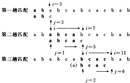
图 4.4 改进算法的匹配过程示例
