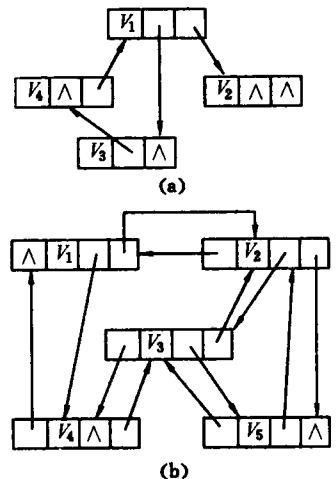
图 7.7 图的多重链表 (a) G_1 的多重链表; (b) G_2 的多重链表
