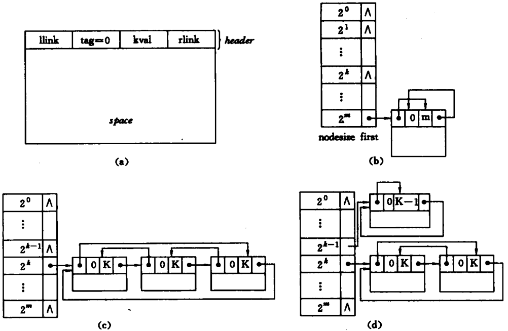
图 8.8 伙伴系统中的可利用空间表 (a) 空闲块的结点结构; (b) 表的初始状态; (c) 分配前的表; (d) 分配后的表
