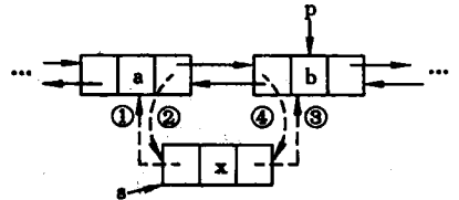
图 2.16 在双向链表中插入一个结点时指针的变化状况
