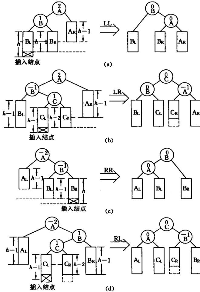
图 9.13 二叉排序树的平衡旋转图例 (a) LL 型; (b) LR 型; (c) RR 型; (d) RL 型
