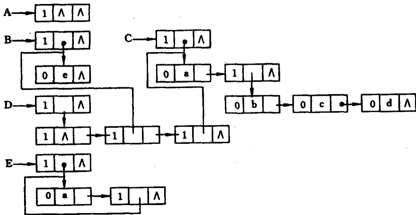
图 5.11 列表的另一种链表表示
