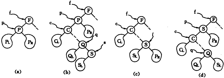
图 9.9 在二叉排序树中删除 * p (a) 以 * f 为根的子树; (b) 删除 * p 之前; (c) 删除 * p 之后,以 P_R 作为 * s 的右子树的情形; (d) 删除 * p 之后,以 * s 替代 * p 的情形
