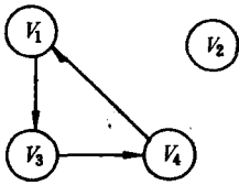
图 7.4 G_1 的两个强连通分量
