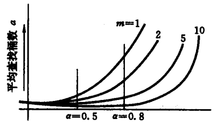
图 12.14 桶的容量和查找次数的关系
