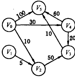
图 7.34 带权有向图 G_5
