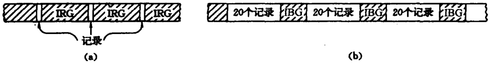
图 11.2 磁带上信息存放示意图 (a) 字符组长 80 字符的磁带；(b) 成块存放的磁带
