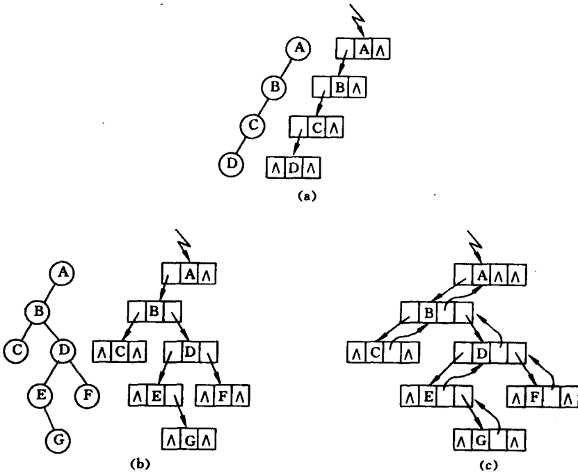
图 6.8 链表存储结构 (a) 单支树的二叉链表; (b) 二叉链表; (c) 三叉链表
