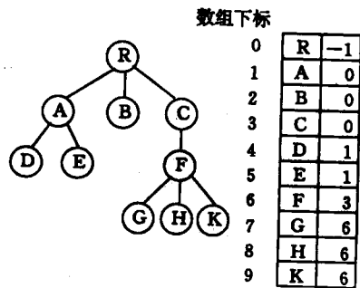
图 6.13 树的双亲表示法示例
