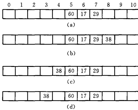
图 9.25 用开放定址处理冲突时,关键字为 38 的记录插入前后的哈希表 (a) 插入前;(b) 线性探测再散列;(c) 二次探测再散列;(d) 伪随机探测再散列,伪随机数列 9,...
