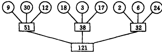
图 11.8 3-路平衡归并的归并树
