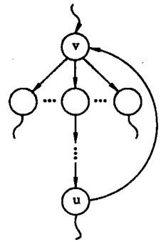
图 7.24 含有环的有向图的深度优先生成树
