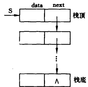
图 3.3 链栈示意图
