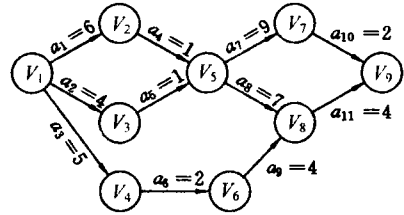
图 7.29 一个 AOE-网
