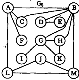
图 7.19 连通图 G_5
