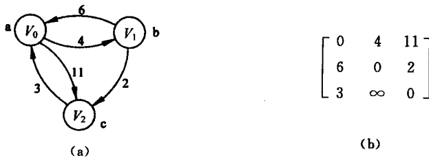
图 7.36 带权有向图
