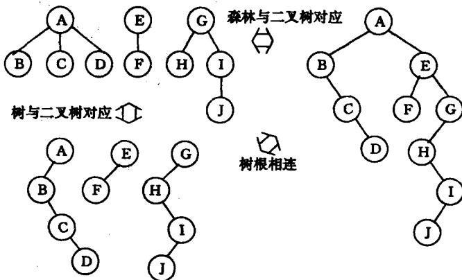
图 6.17 森林与二叉树的对应关系示例
